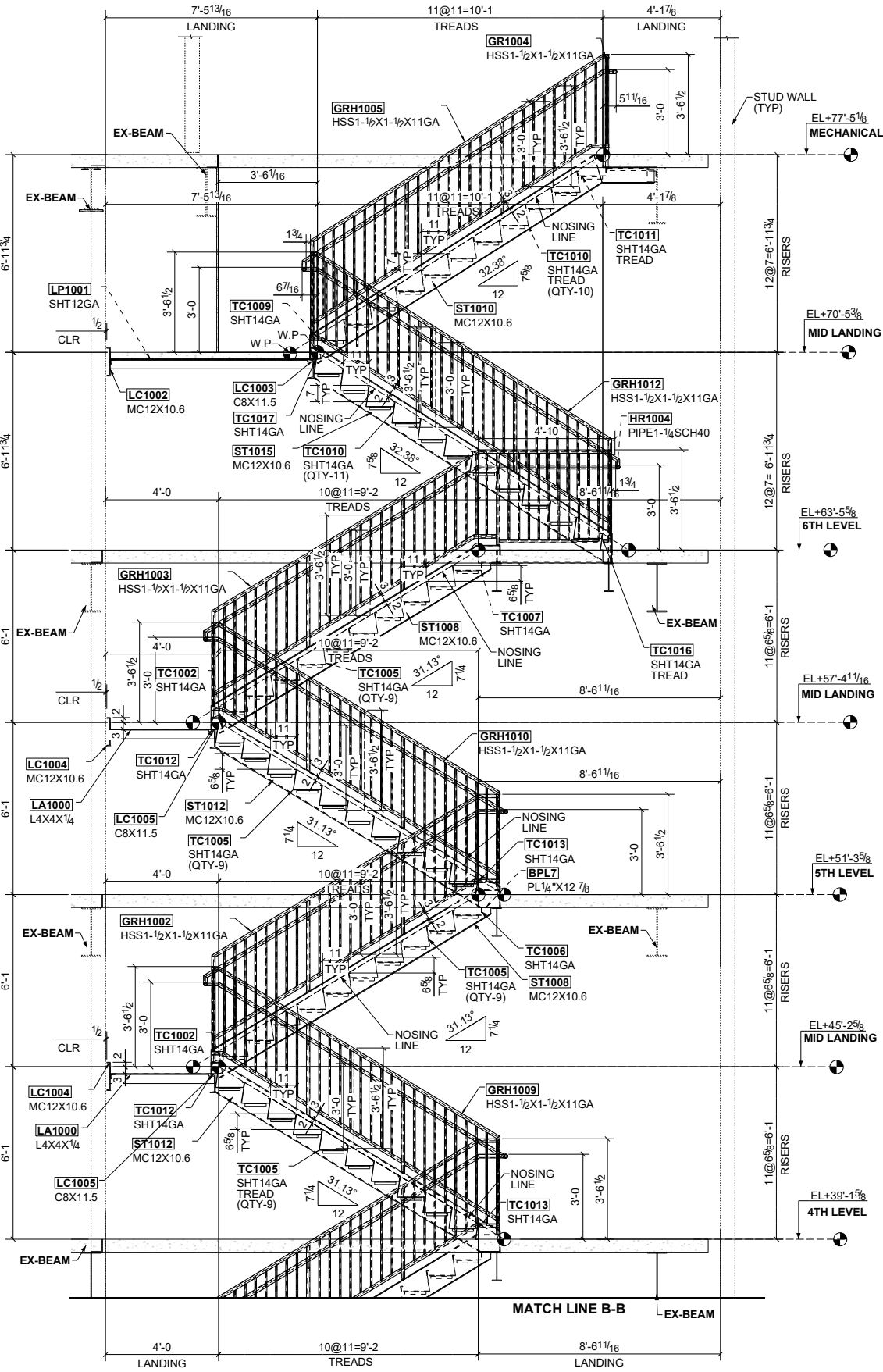
B ELEVATION VIEW (REF.DWG.NO:4/A7.01) SCALE: 1:28
