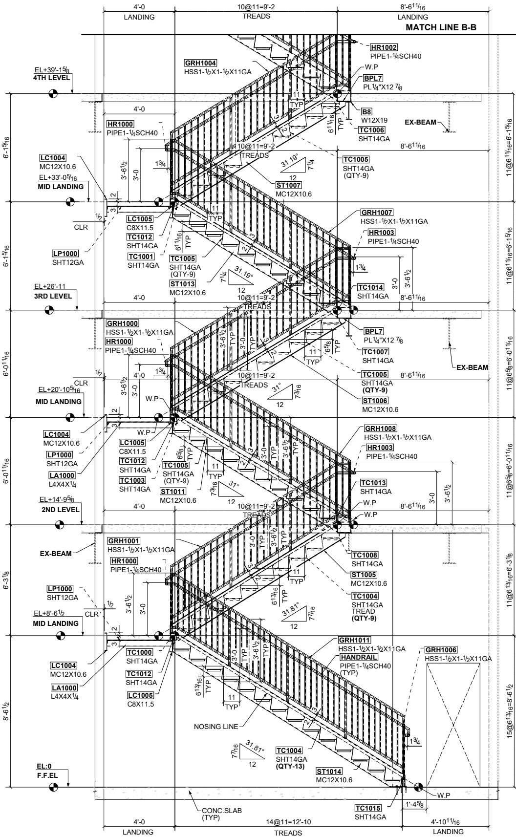
B ELEVATION VIEW (REF.DWG.NO:4/A7.01) SCALE: 1:28
