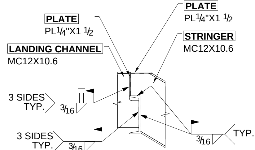
SECTION E - E
