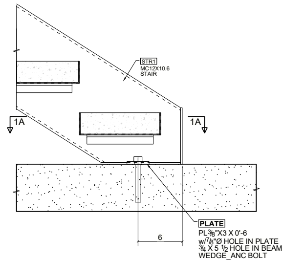
DETAIL - 1 E9
