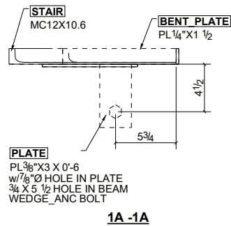
1A - 1A
