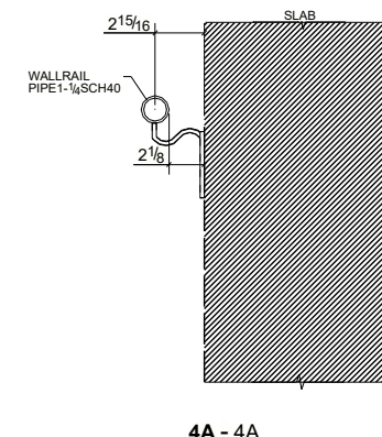
4A - 4A
