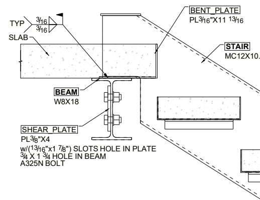
DETAIL-3 E9
