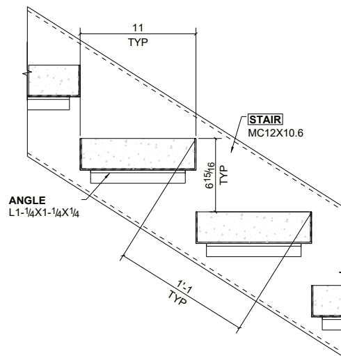
DETAIL 2 E9
